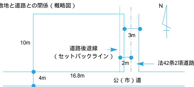
敷地と道路との関係 (概略図)
